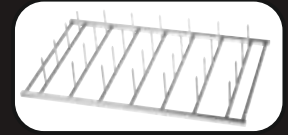
Στηρίγματα για πατάτες Διάσταση : GN 2/3
