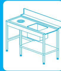
Πάσο εισόδου πλυντηρίου με 1 γούρνα 50 x 40 cm και οπή για απορρίματα (Αριστερό - Δεξί) Διαστάσεις : 180 x 73 x 85 cm Βάρος : 55 Kg
