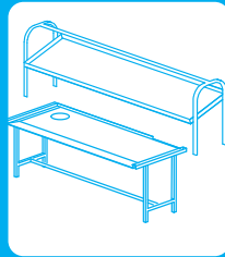
Τραπέζι παραλαβής απλύντων με οπή για απορρίματα + επιτραπέζιο ράφι κανίστρων Διαστάσεις : 240 x 100 x 87 cm Βάρος : 100 Kg
