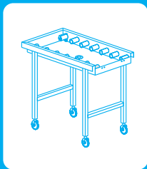
Ραουλοδιάδρομος Διαστάσεις : 164 x 65 x 85 cm Βάρος : 50 Kg
