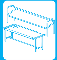
Τραπέζι παραλαβής απλύντων με οπή για απορρίματα + επιτραπέζιο ράφι κανίστρων Διαστάσεις : 160 x 100 x 87 cm Βάρος : 70 Kg
