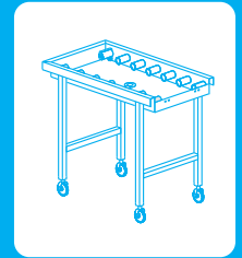
Ραουλοδιάδρομος Διαστάσεις : 114 x 65 x 85 cm Βάρος : 40 Kg
