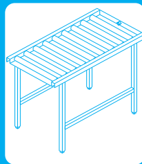
Ραουλοδιάδρομος Διαστάσεις : 160 x 65 x 85 cm Βάρος : 55 Kg
