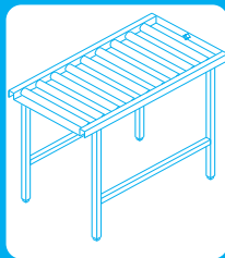
Ραουλοδιάδρομος Διαστάσεις : 110 x 65 x 85 cm Βάρος : 49 Kg
