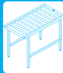
Ραουλοδιάδρομος Διαστάσεις : 210 x 65 x 85 cm Βάρος : 65 Kg
