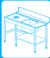
Πάσο εισόδου πλυντηρίου με 1 γούρνα 50 x 40 cm και οπή για απορρίματα (Αριστερό - Δεξί) Διαστάσεις : 120 x 73 x 85 cm Βάρος : 45 Kg
