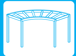
Γωνιακός ραουλοδιάδρομος 90° Διαστάσεις : 130 x 130 x 85 cm Βάρος : 60 Kg
