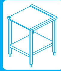
Γωνιακό πάσο πλυντηρίου Διαστάσεις : 59 x 59 x 85 cm Βάρος : 20 Kg
