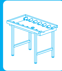
Ραουλοδιάδρομος Διαστάσεις : 160 x 65 x 85 cm Βάρος : 50 Kg
