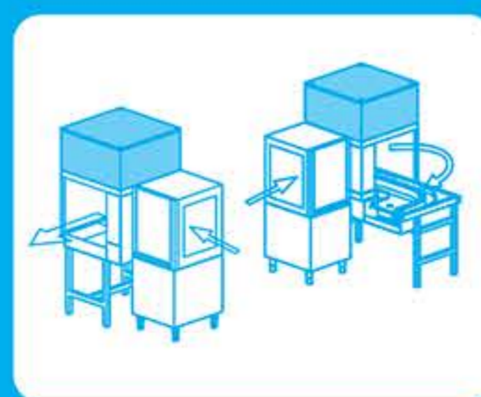
Θάλαμος στεγνώματος (Γωνία 90 °) Ισχύς: 6 Kw Διαστάσεις: 85 x 85 x 185 cm
