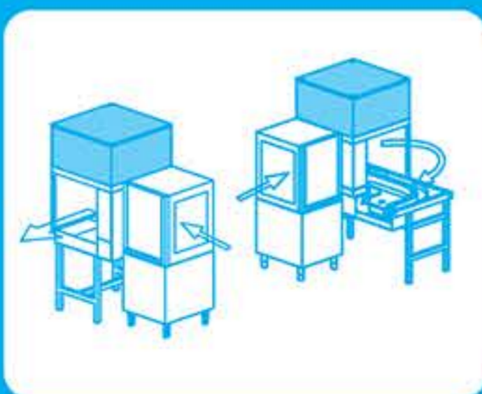
Θάλαμος στεγνώματος (Γωνία 90 °) με μοτέρ για την κίνηση των κανίστρων Ισχύς: 12 Kw Διαστάσεις: 85 x 85 x 195 cm
