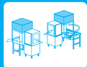
Θάλαμος στεγνώματος (Γωνία 90 °) με μοτέρ για την κίνηση των κανίστρων Ισχύς: 12 Kw Διαστάσεις: 85 x 85 x 195 cm
