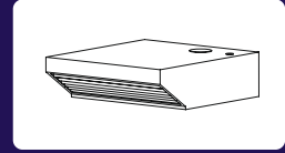
Απορροφητήρας - Καπέλο Διαστάσεων: 92 x 99 x 30 cm Ισχύς: 0,25 Kw Τάση: 230 V
