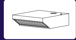
Απορροφητήρας - Καπέλο Διαστάσεων: 99 x 115 x 30 cm Ισχύς: 0,25 Kw Τάση: 230 V
