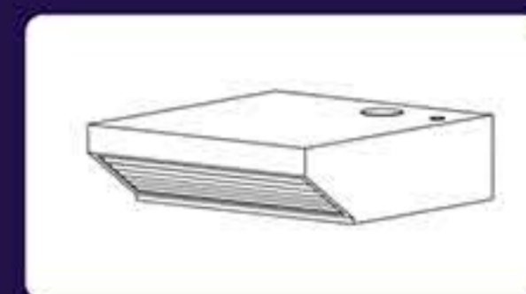
Απορροφητήρας - Καπέλο Διαστάσεων: 83 x 83 x 30 cm Ισχύς: 0,25 Kw Τάση: 230 V
